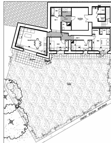
Plan d'ensemble
