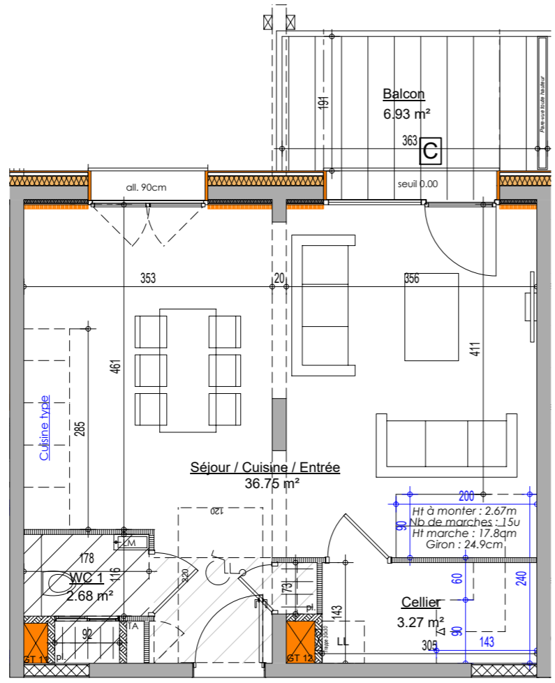
Niveau BAS
